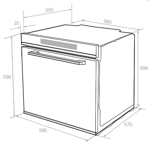
Dimensions d'encastrement Built in Dimensions
